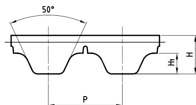
ATL5 - ATL10 - ATL20
