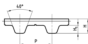
L - H - XH
