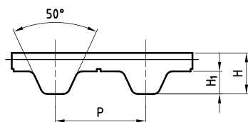
L - H - XH
