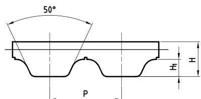
AT5 - AT10 - AT20
