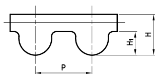
HTD8M TP
